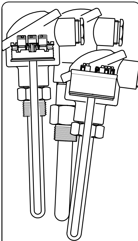
capteurs à tête de raccordement avec élément de mesure interchangeable
